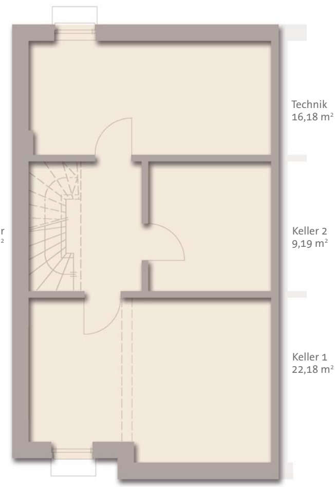
Kellergeschoss
